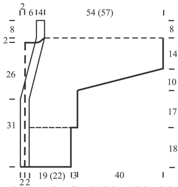
Linkes Vorderteil und Rückenteil (Jacke) Left front and back (cardigan)
